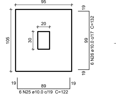
S7 PLANTA ESC 1:25
