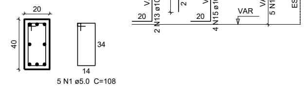
P1 FUNDACAO - L1 ESC 1:20
