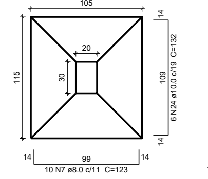
S6 PLANTA ESC 1:25
