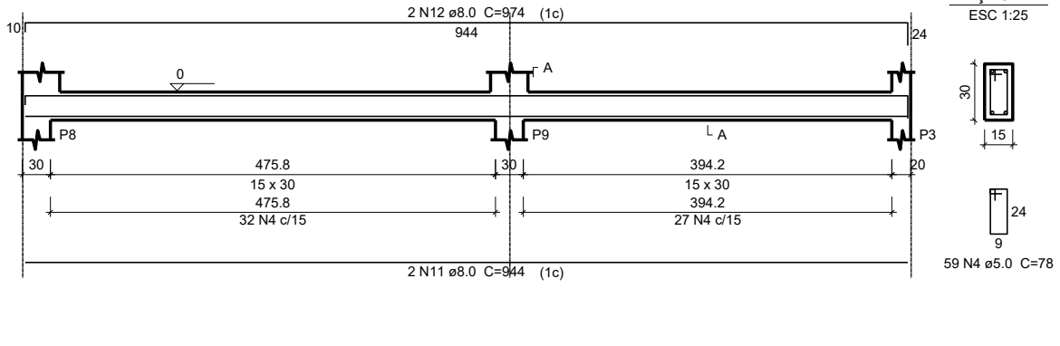
V2 ESC 1:50
