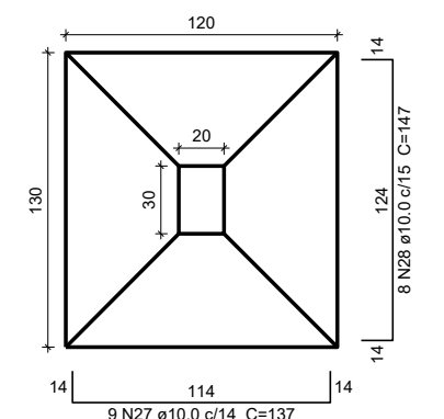
S8 PLANTA ESC 1:25
