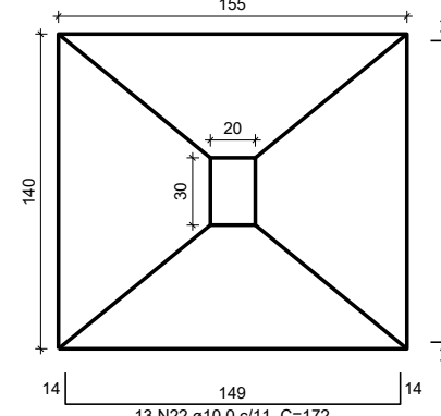
S4 PLANTA ESC 1:25
