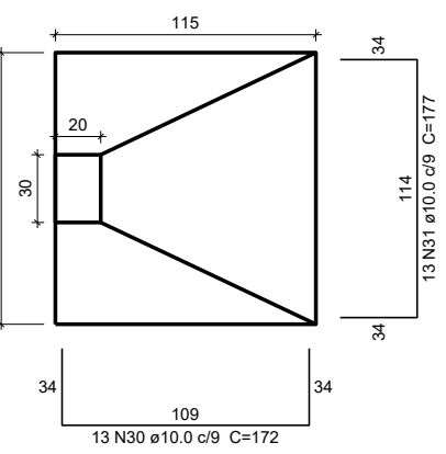
S9 PLANTA ESC 1:25
