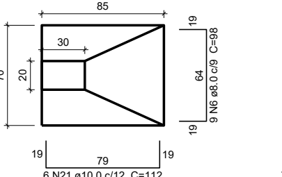
S3 PLANTA ESC 1:25
