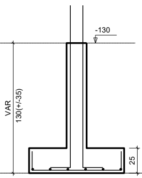
CORTE ESC 1:25
