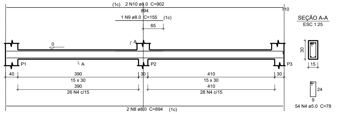
V1 ESC 1:50
