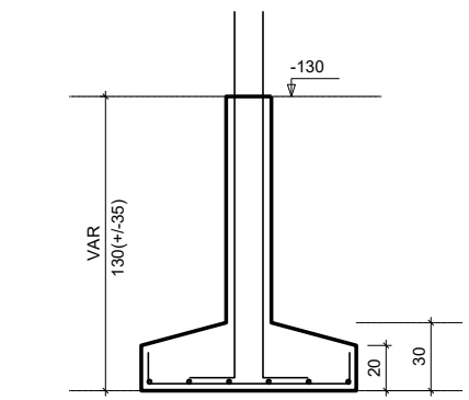
CORTE ESC 1:25
