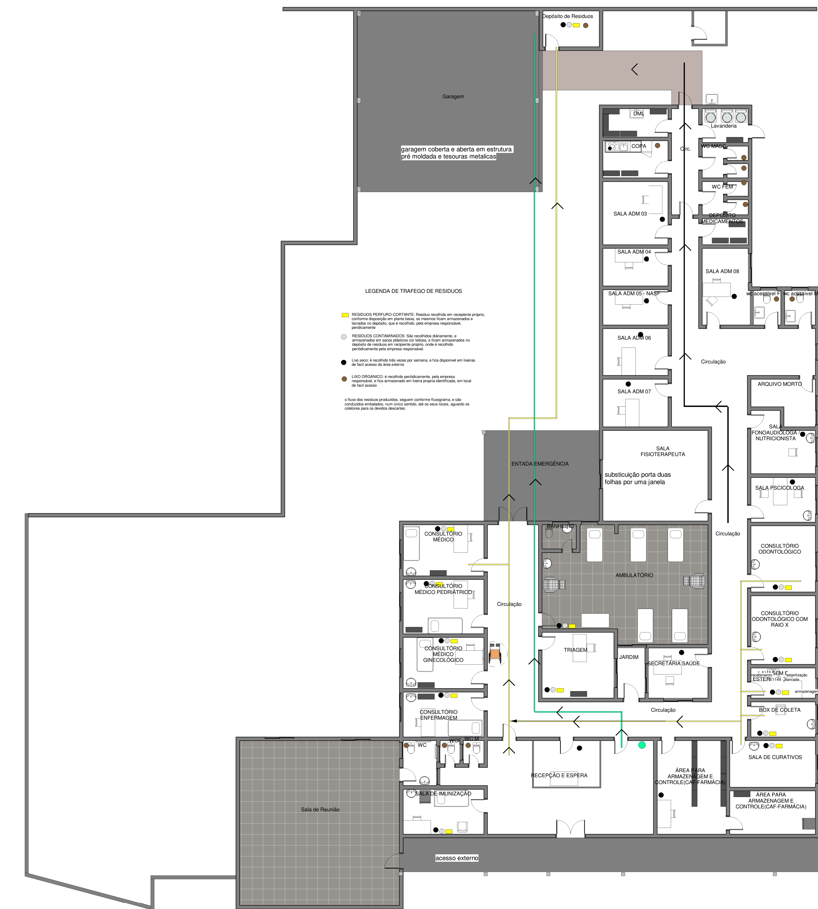
1 PLANTA BAIXA FLUXOGRAMA 1 : 100
